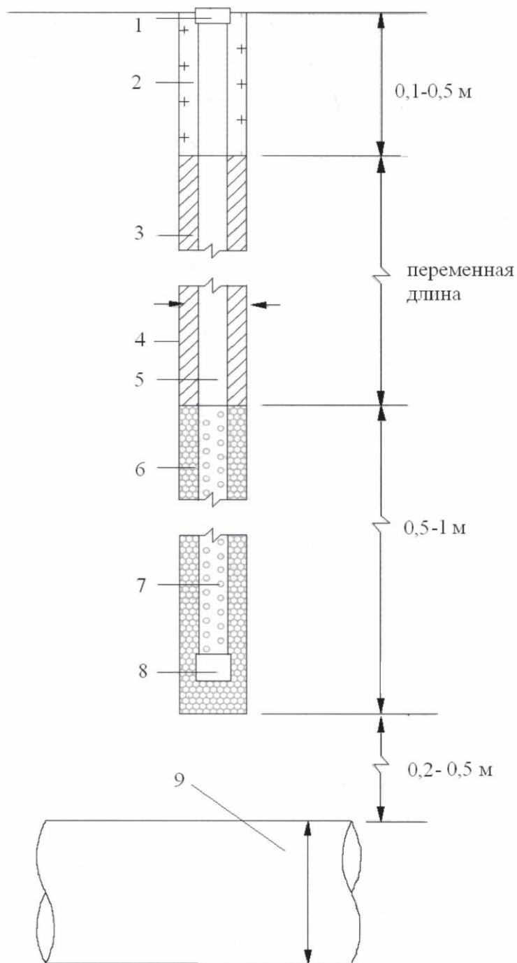
1 – заглушка с вентиляционным отверстием; 2 – грунтовая засыпка; 3 – заполнение тампонажным глиноцементным раствором; 4 – ствол скважины диаметром 200 мм; 5 – ПВХ-труба диаметром от 75 до 100 мм; 6 – гравийная засыпка от 0,5 до 1,0 м; 7 – перфорированный фильтр; 8 – водонепроницаемая заглушка; 9 – буровой ствол скважины ГНБ после расширения Рисунок 8.2 - Схема разгрузочной скважины.
