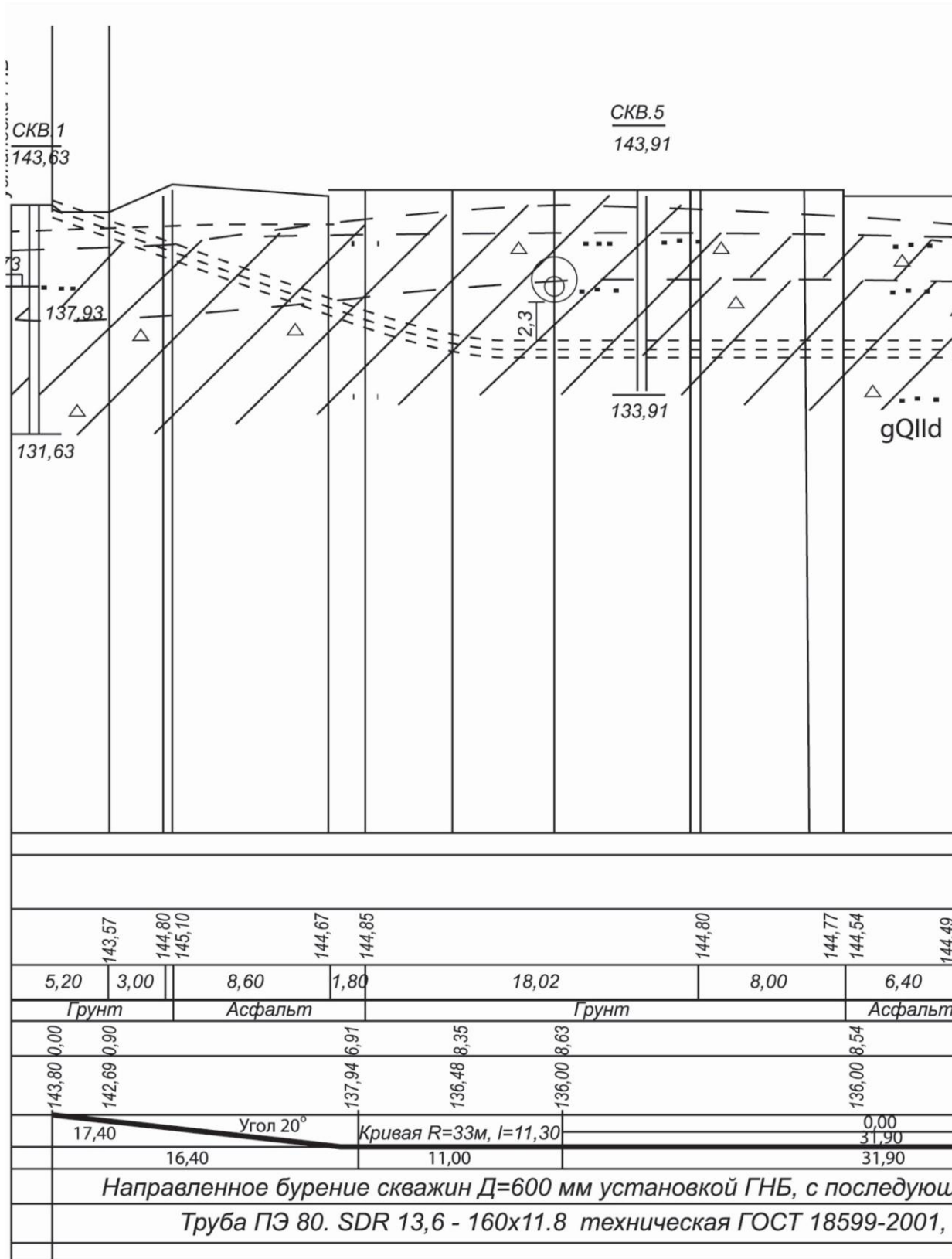
7.1 – Пример построения продольного профиля
